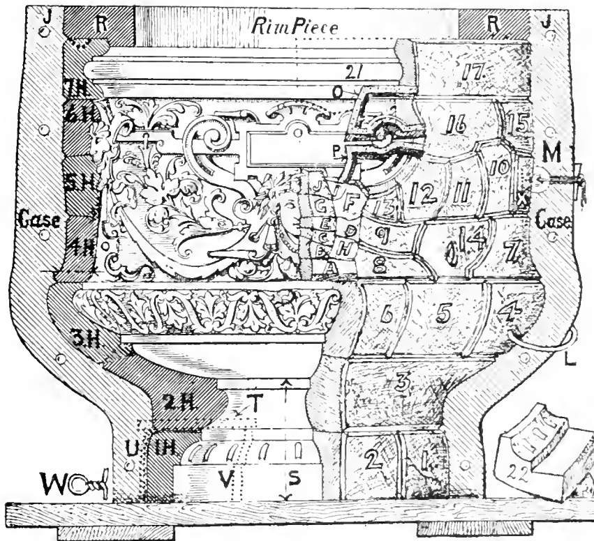
NO. 95.—PLASTER PIECE MouldING VASE.
